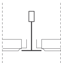
BANDEJA CAPRI ENRASADA (T-24)
