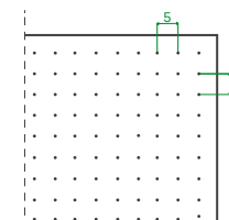
Perforado Ø 0,7 U | 2% perforado
