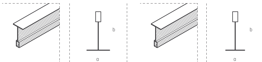
PERFIL T-24 X 38
