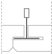
PERFIL OCULTO DESMONTABLE P5S
