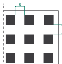
Perforado 8x8 24% perforado
