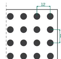
Perforado Ø6 17% perforado
