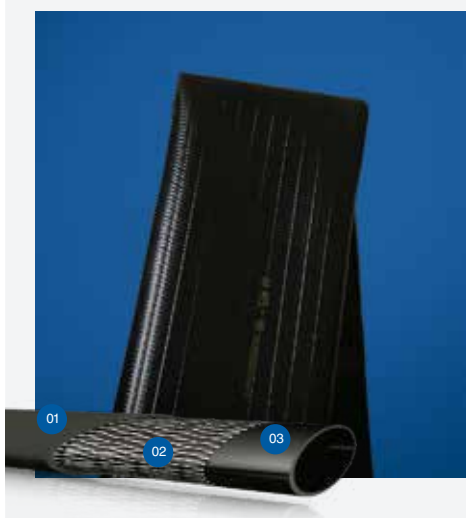
01.-Elastómero nitrilo. 02.-Refuerzo con hilo de poliéster de alta tenacidad. 03.-Elastómero nitrilo.
