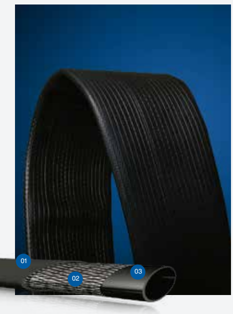
01.-Elastómero nitrilo. 02.-Reforzado con hilo de poliéster de alta tenacidad. 03.-Elastómero nitrilo.
